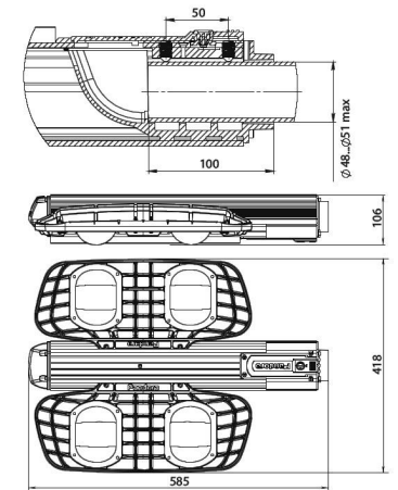
Рисунок 3. Габаритный чертеж
